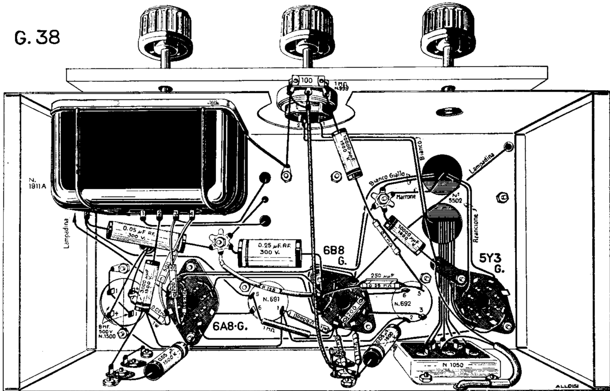
Piano di costruzione.
